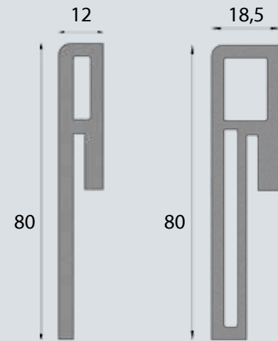
Kompozit Süpürgelik / Composite Plinths
